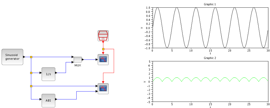
Рис. 8. Использование CMSCOPE
