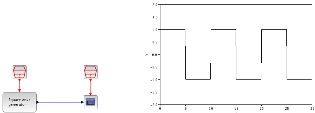
Рис. 11. Использование GENSQR_f
