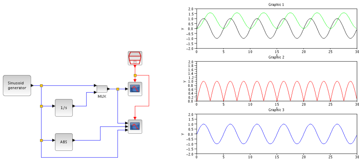
Рис. 9. Расширенное использование CMSCOPE
