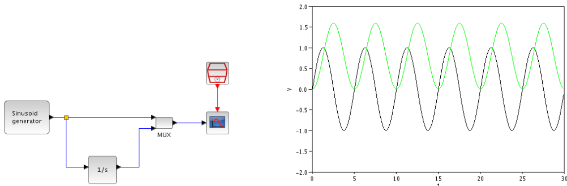
Рис. 7. Использование CSCOPE
