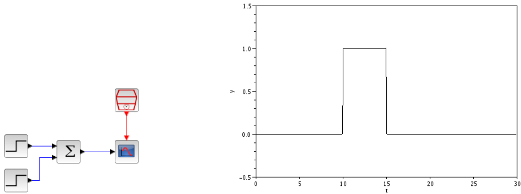
Рис. 15. Одиночный прямоугольный импульс
