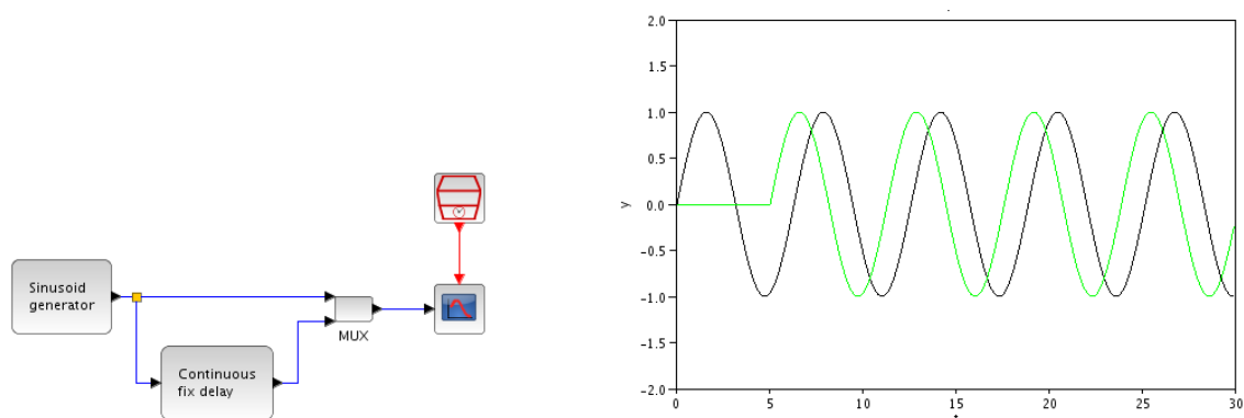
Рис. 18. Использование блока задержки
