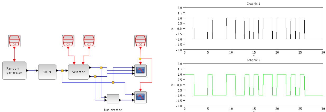
Рис. 17. Использование шины
