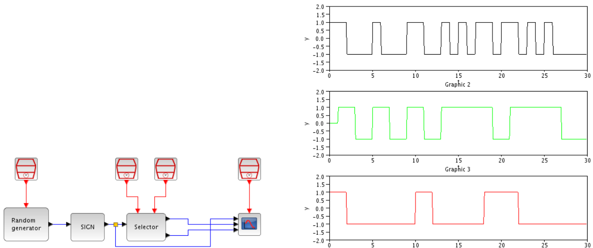
Рис. 16. Использование селектора
