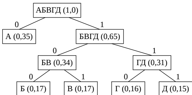
Рис. 2. Кодовое дерево кода Хаффмана
