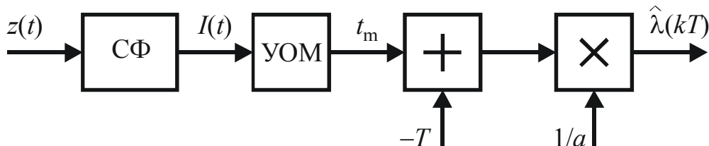
Рис. 4. Оценитель параметра \lambda при ВМ
