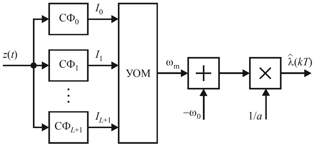
Рис. 3. Схема оценителя частоты с использованием согласованных фильтров
