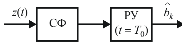
Рис. 6. Схема демодулятора сигнала ФМ-2 на согласованном фильтре
