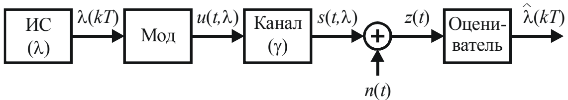
Рис. 1. Структурная схема системы передачи параметра \lambda в аналоговой форме
