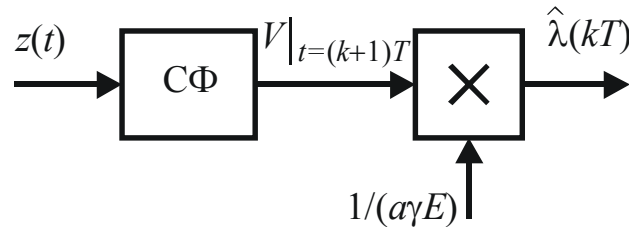
Рис. 2. Структурная схема оценителя амплитуды
